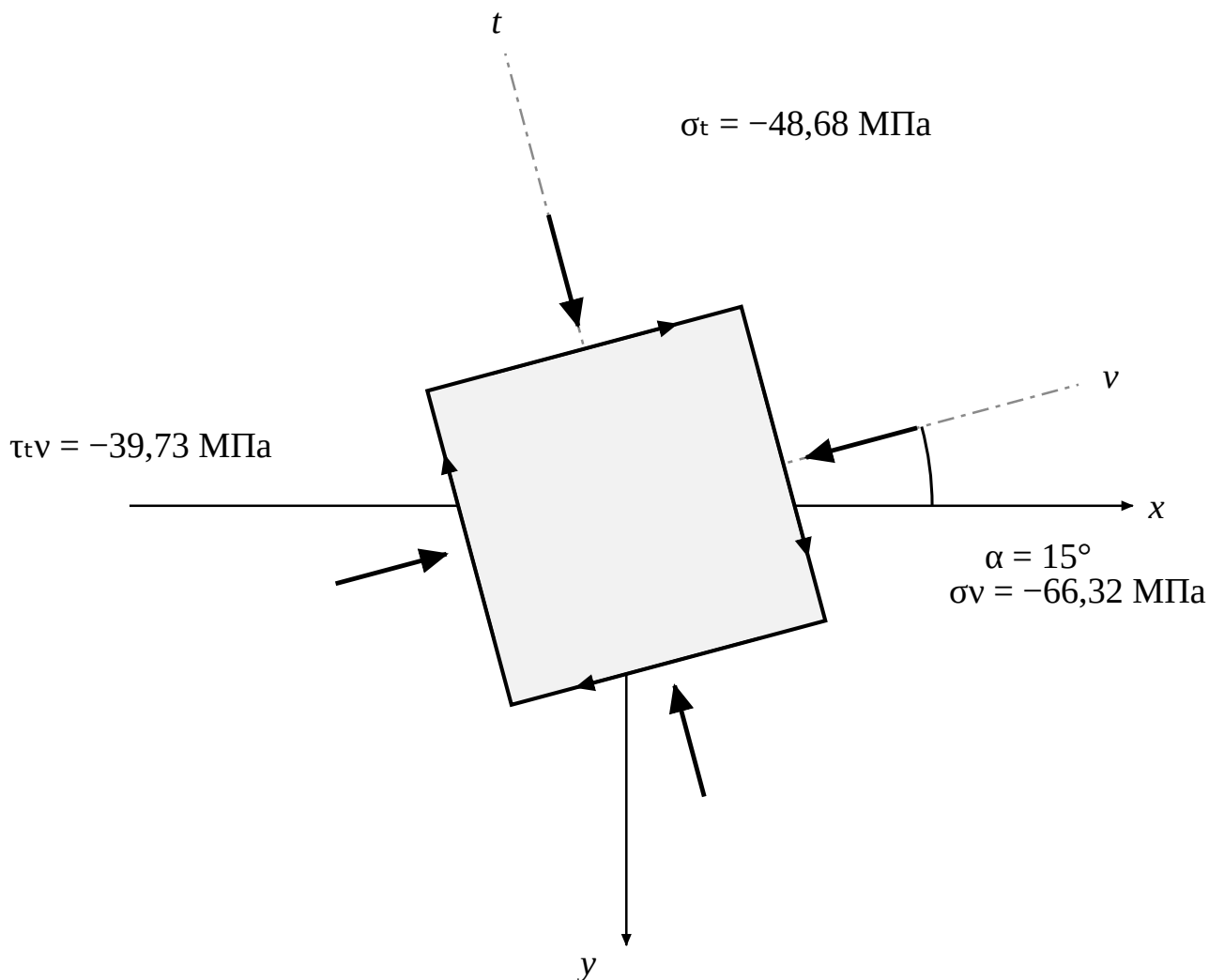
Рис. 2.5 — напряжения на площадках, повёрнутых на \alpha = 15^\circ . Оба нормальных напряжения сжимающие, стрелки направлены к граням; касательные образуют уравновешенную пару.
