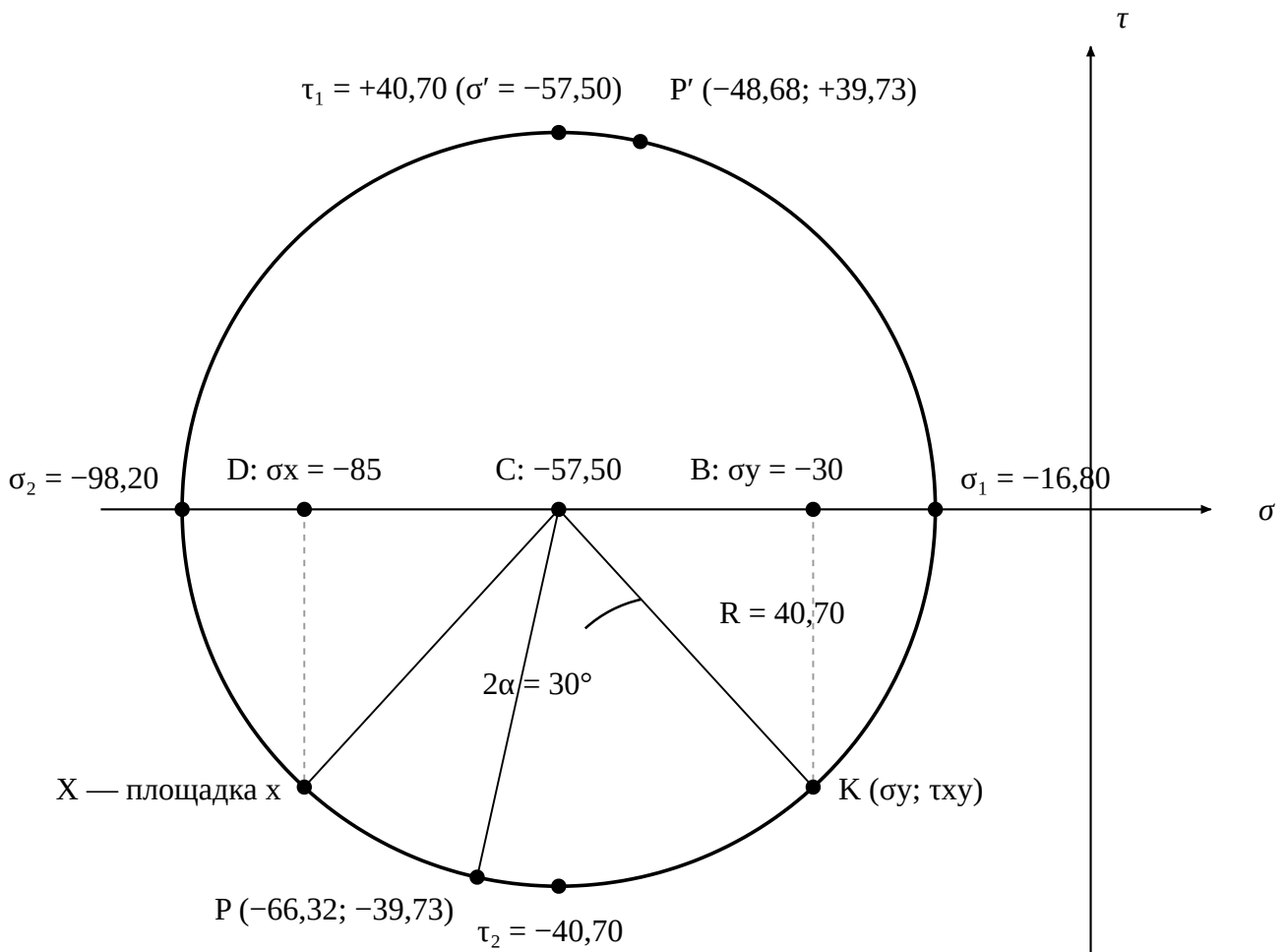
Рис. 2.6 — круг Мора. Построение: D и B — исходные \sigma_x и \sigma_y на оси; C — центр; BK = \tau_{xy} отложено от B вниз; R = CK . С круга снимаются \sigma_1 и \sigma_2 (пересечения с осью), \tau_1 и \tau_2 (верх и низ), точка P — площадка под \alpha = 15^\circ , P' — перпендикулярная ей. Все шесть величин совпали с аналитическим расчётом.
